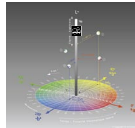
ESPACE CIE 1976 Repérage en coordonnées cylindriques L* C* h
